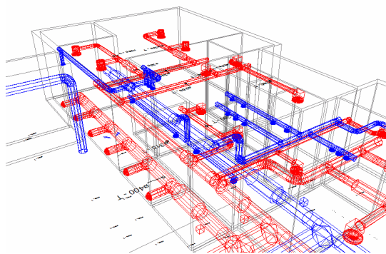
3D perspektiv av balansert ventilasjon
